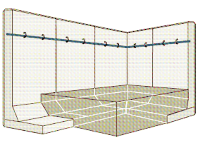
Przykład uformowania narożnika z prętami okrągłymi \phi 16 mm i nadbetonem C 16/20
