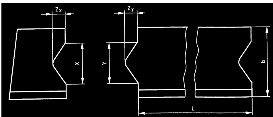
Rys.1. Przykład kształtu krawężnika przeznaczonego do ryglowania
