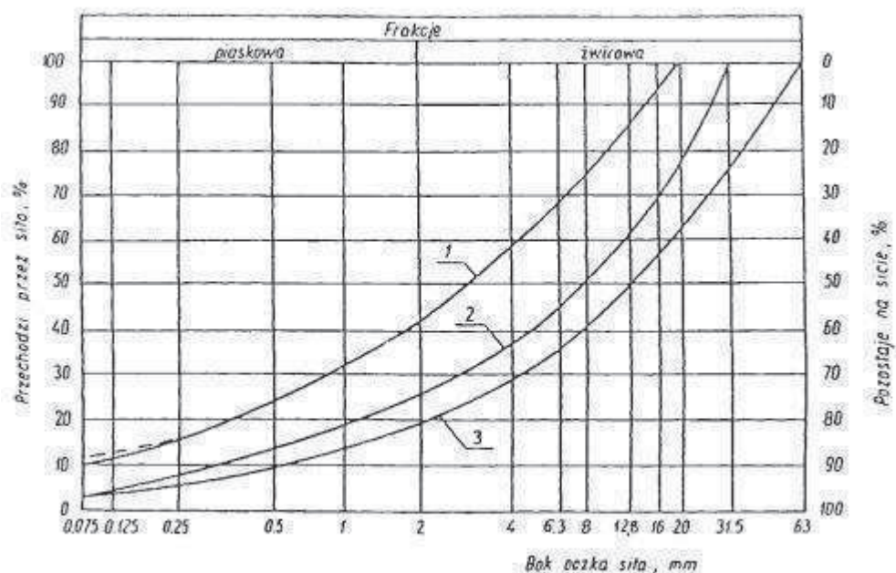
Rysunek 1. Pole dobrego uziarnienia kruszywa na podbudowę muru oporowego - linie 1-2
