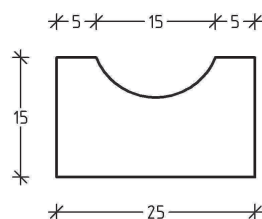
Rys. 1. Betonowy ściek prefabrykowany
