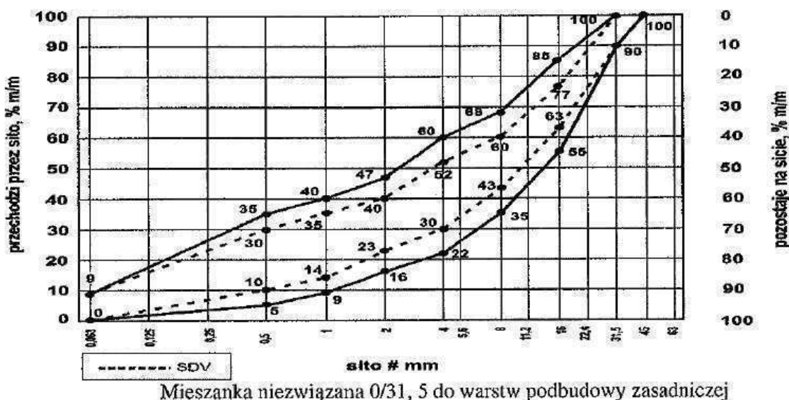
Rys. nr 1 Krzywe uziarnienia mieszanki
