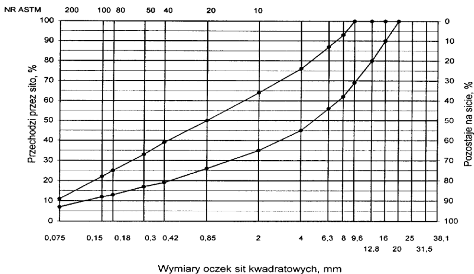
Rys. 1. Krzywe graniczne uziarnienia mieszanki mineralnej BA 0 do 12,8 mm do warstwy ścieralnej nawierzchni drogi o obciążeniu ruchem KR 1- KR 2
